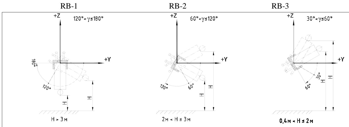
Рис. 3. Наклон пассажирских кресел набор
